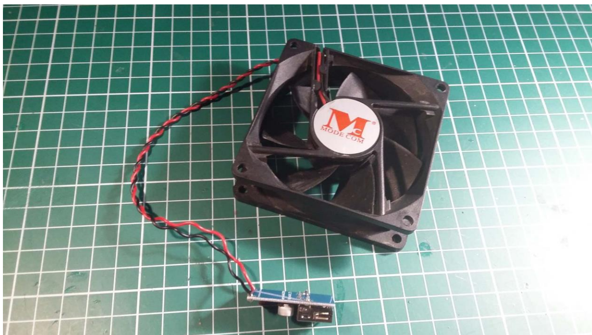
Fot. 43. Wentylator z przylutowaną przetwornicą step-up
