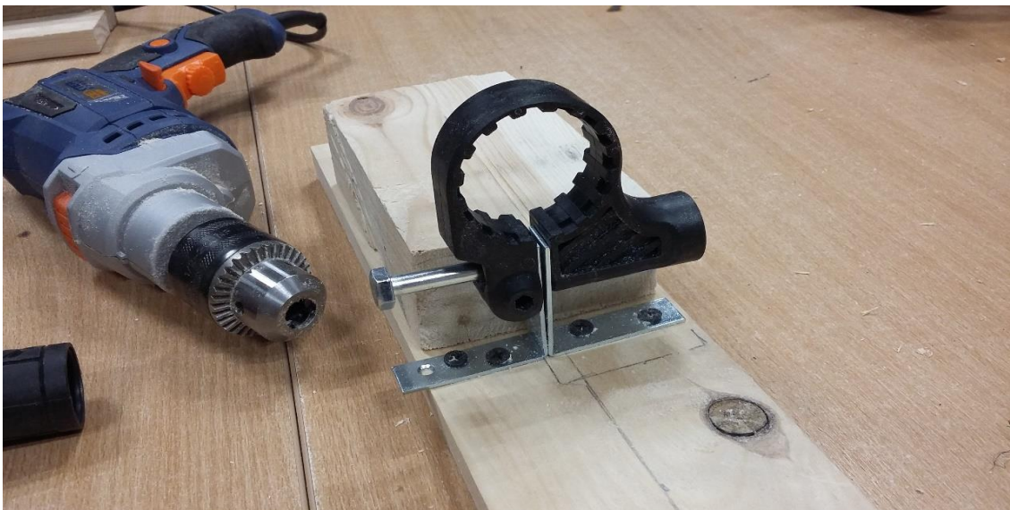
Fot.31. Uchwyt wiertarski – montaż – etap pierwszy
