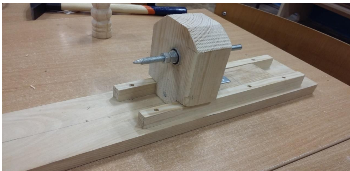
Fot. 33. Konik tokarki
