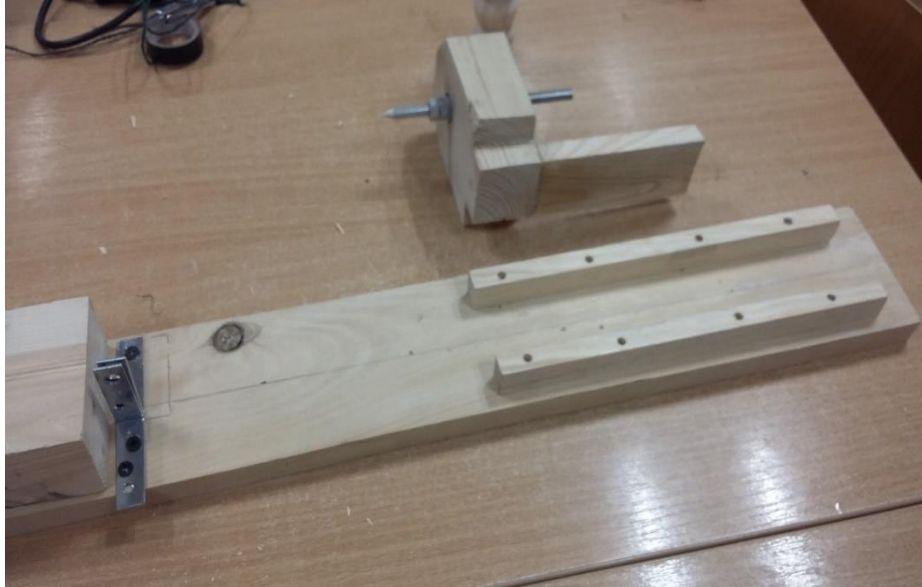
Fot. 38. Mocowanie listewek- prowadnic, które będą utrzymywały konik w osi
